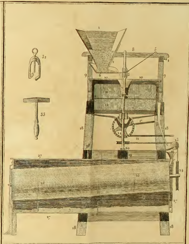
COUPE VERTICALE.
