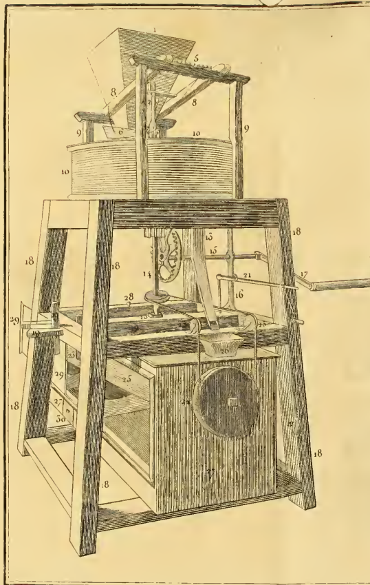
du Moulin à bras inventé par le Cit. DURAND Père et Fils.
